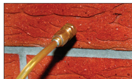
Naniesienie produktu BOTAMENT ® MS 80 W metodą natryskową
